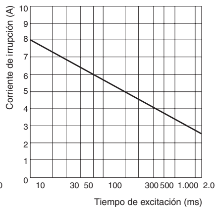
G3R-ODX02SN-UTU
